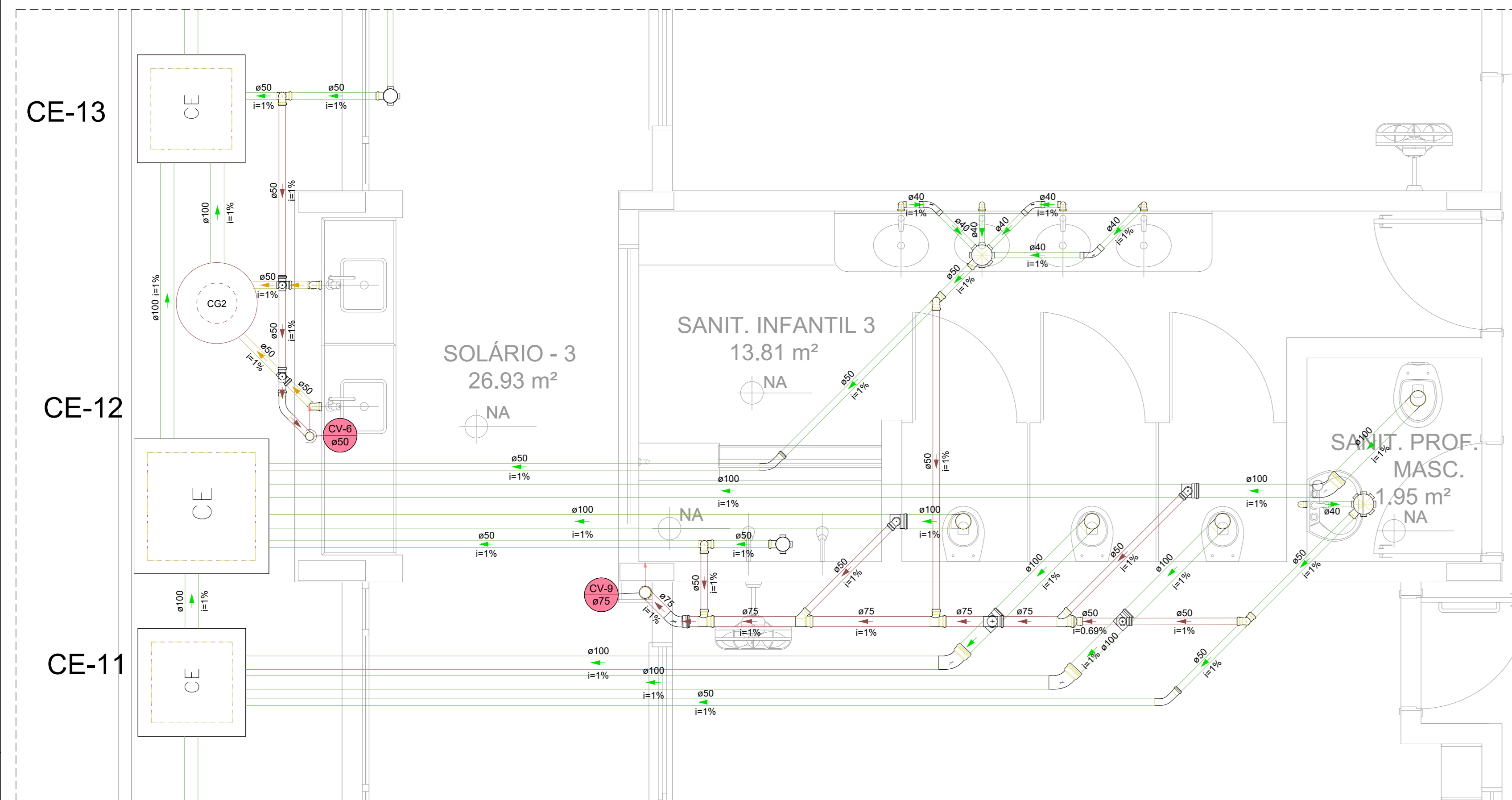
Detalhe SAN-4 Escala 1:25
