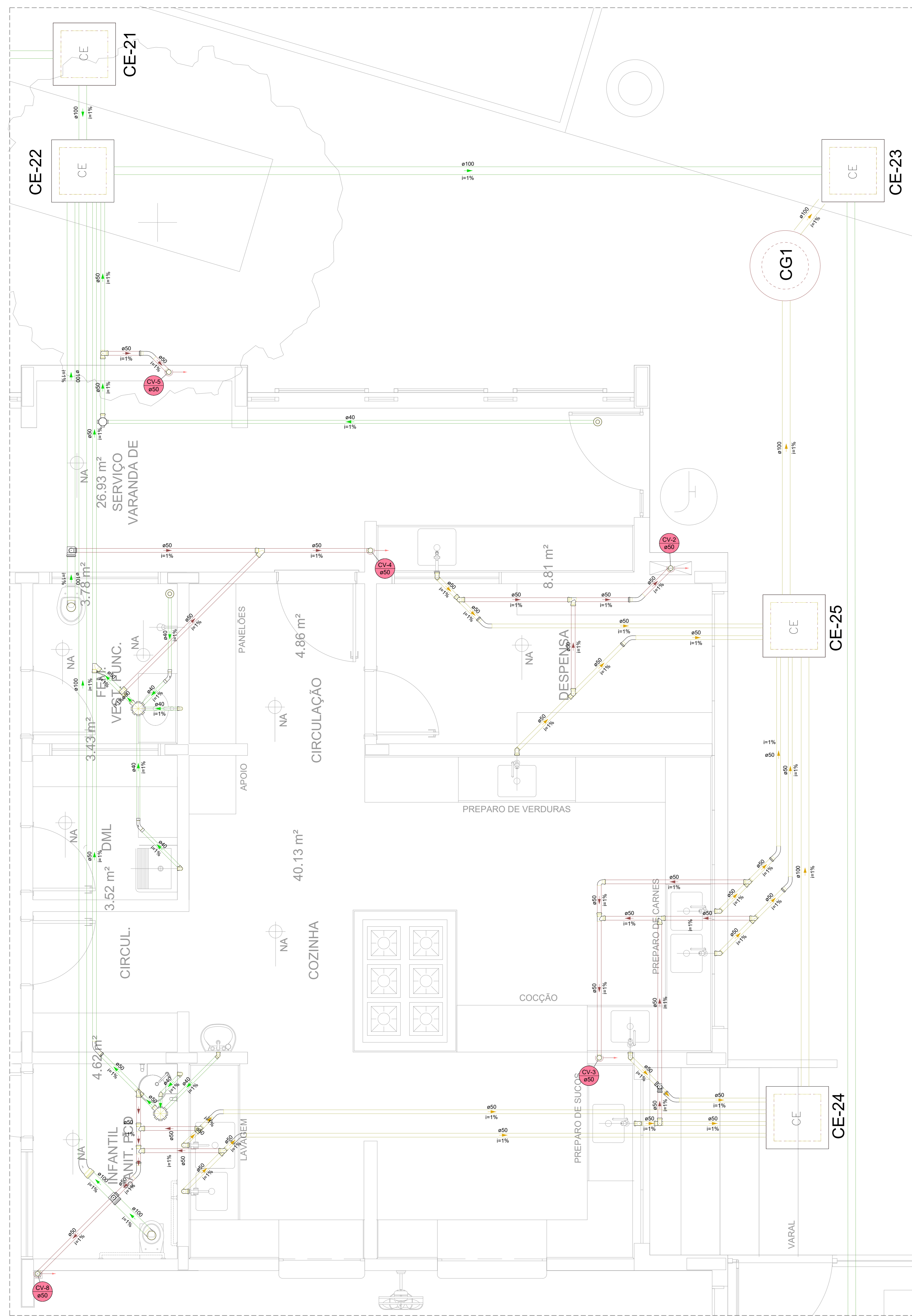
Detalhe SAN-15 Escala 1:25
