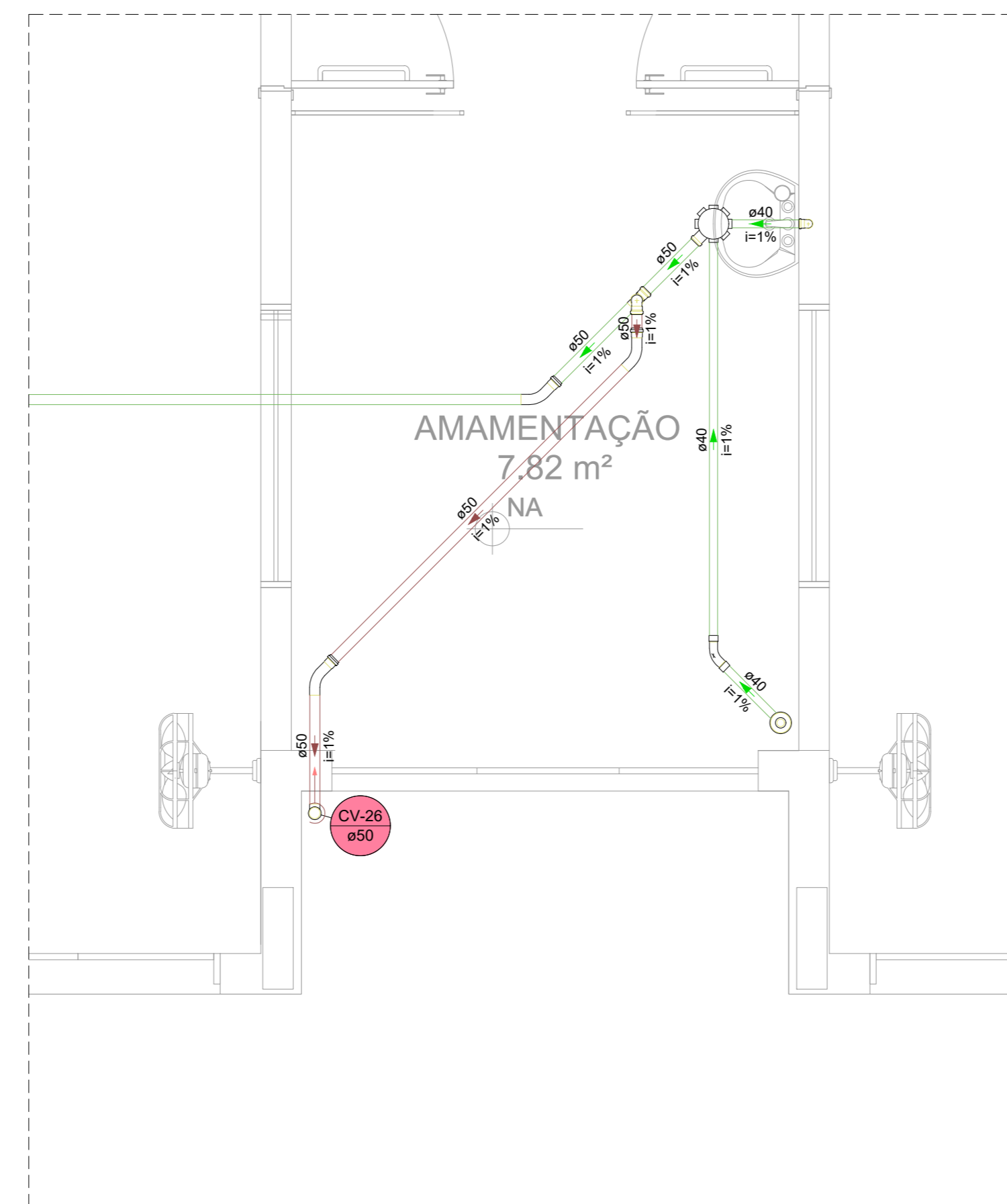
Detalhe SAN-13 Escala 1:25
