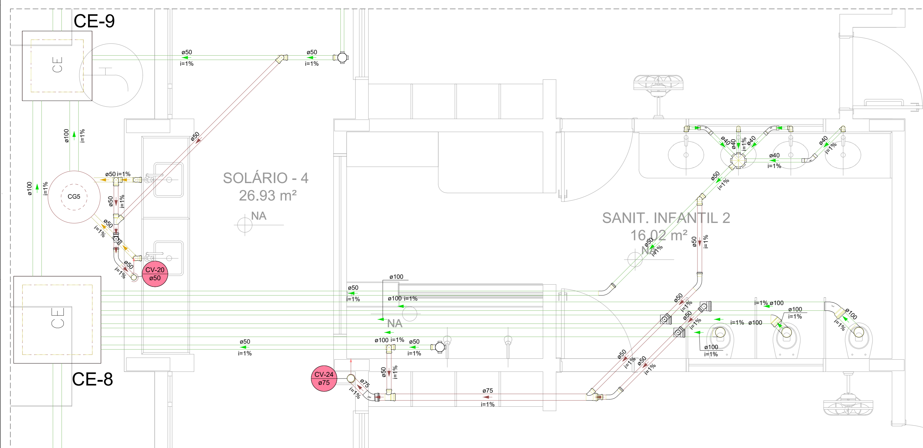
Detalhe SAN-10 Escala 1:25
