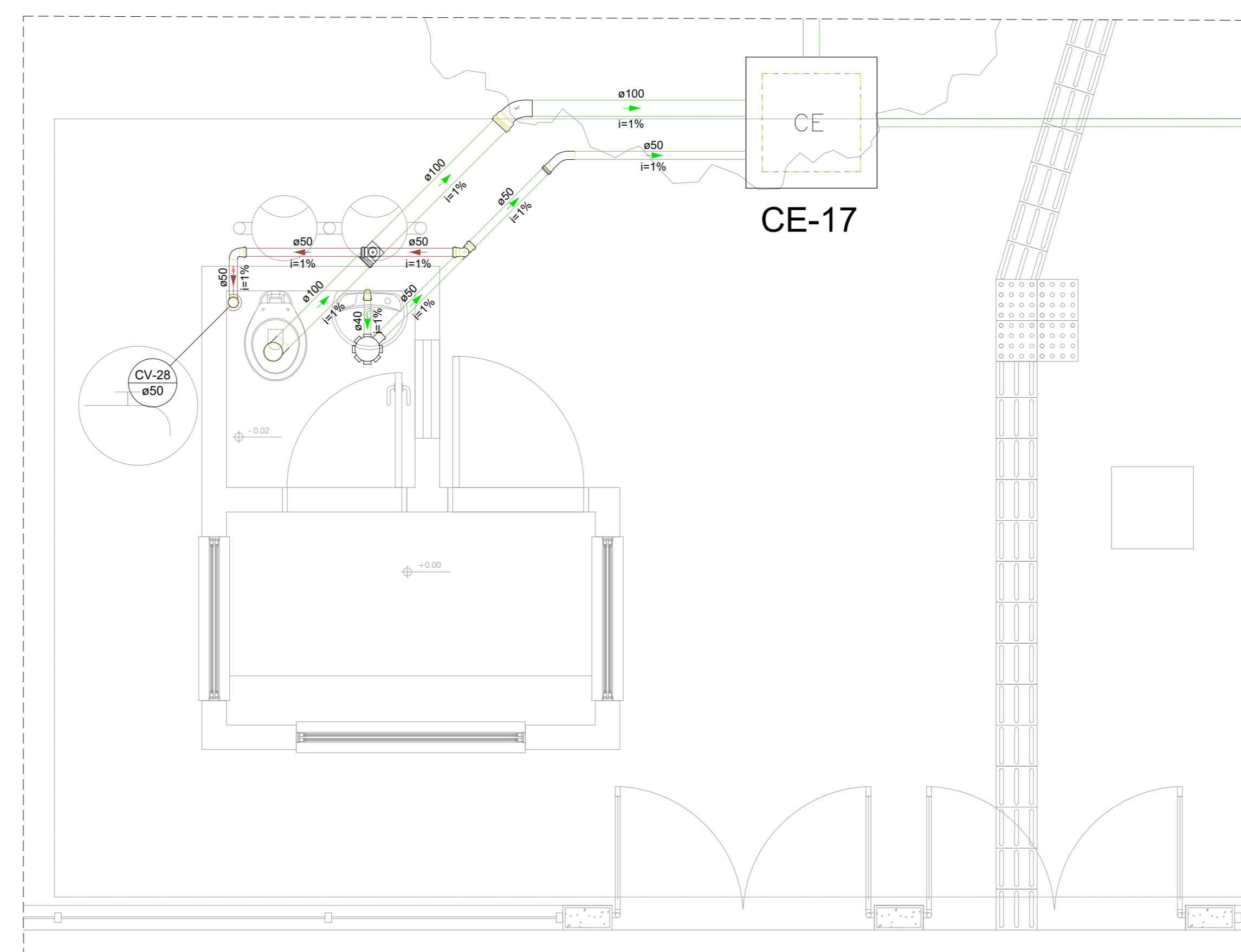
Detalhe SAN-14 Escala 1:25
