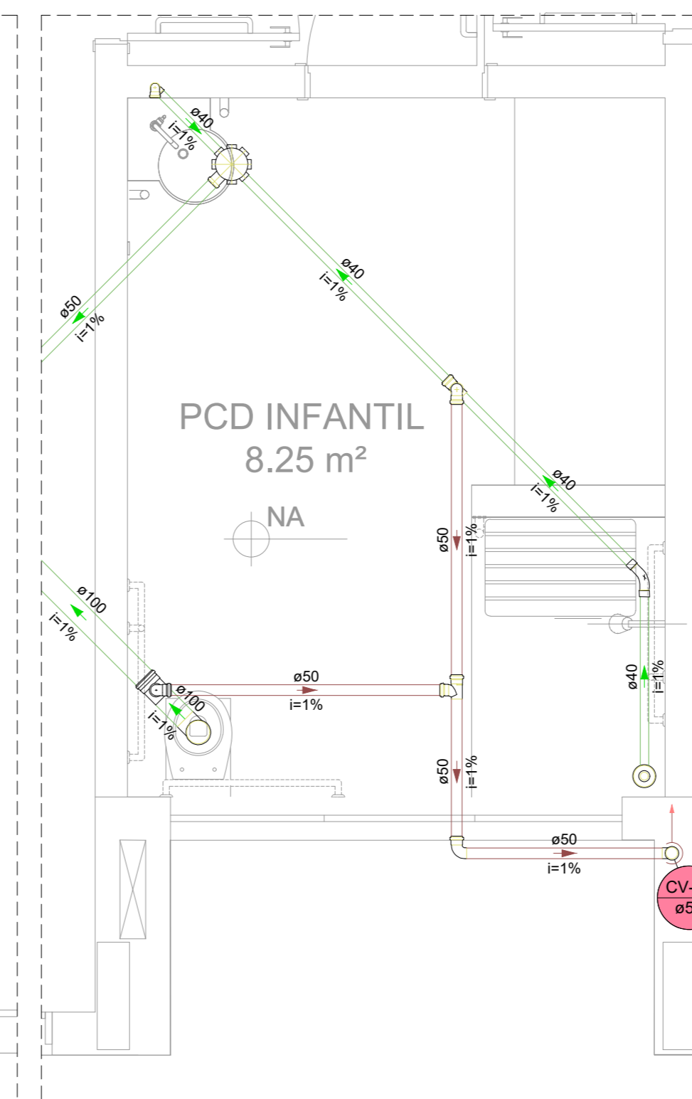
Detalhe SAN-12 Escala 1:25
