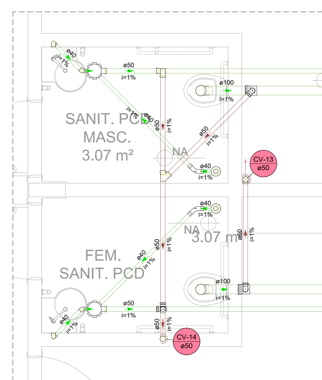
Detalhe SAN-7 Escala 1:25
