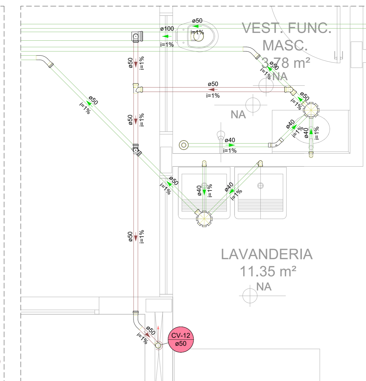
Detalhe SAN-5 Escala 1:25
