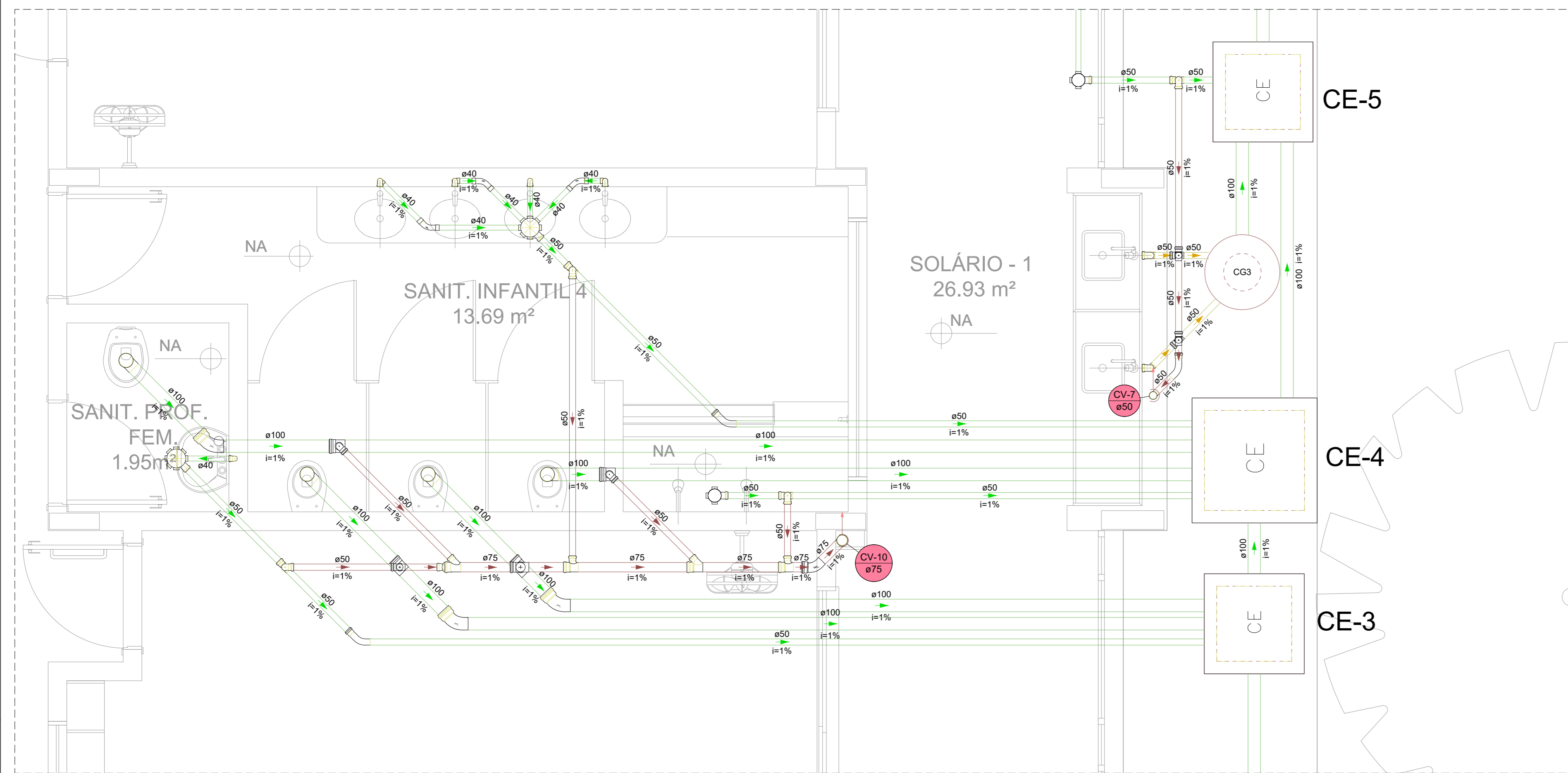
Detalhe SAN-3 Escala 1:25
