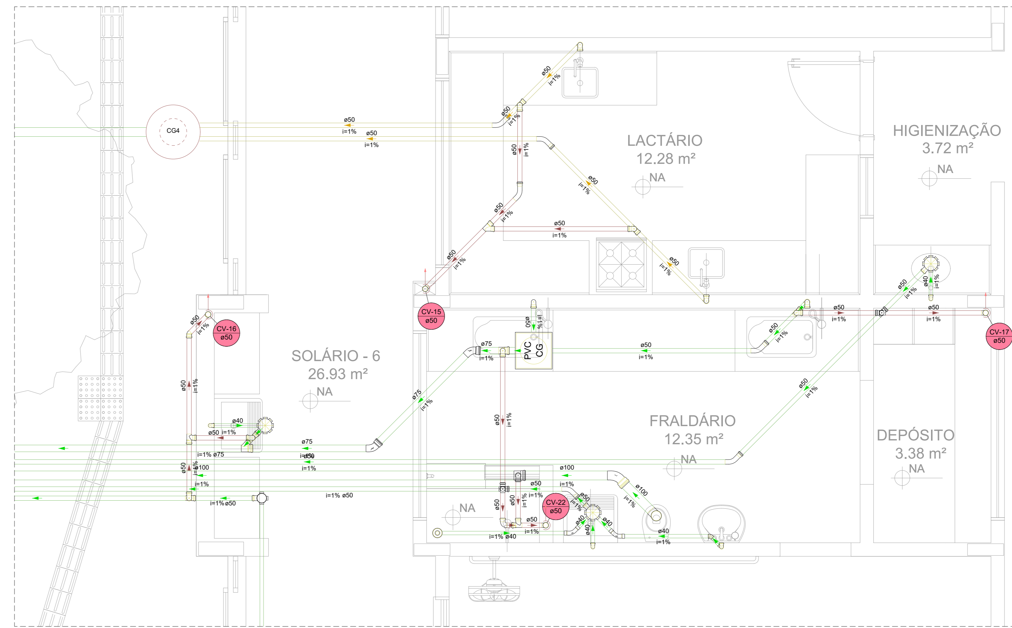
Detalhe SAN-8 Escala 1:25
